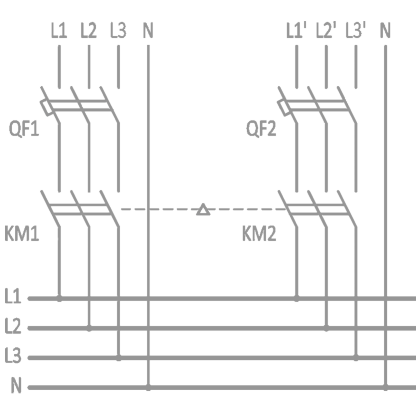
СХЕМА 3. ТРЕХФАЗНЫЙ АВР
