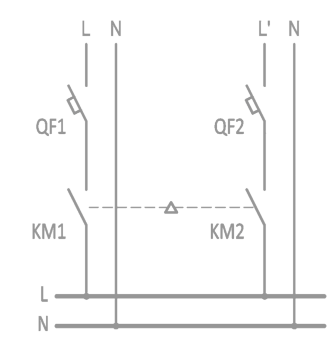
СХЕМА 1. ОДНОФАЗНЫЙ АВР
