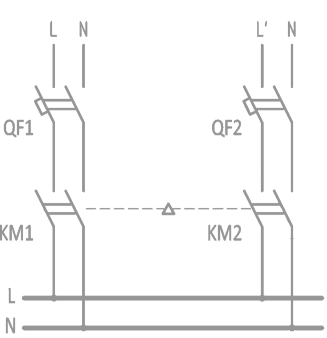
СХЕМА 2. ОДНОФАЗНЫЙ АВР С КОММУТАЦИЕЙ НЕЙТРАЛИ
